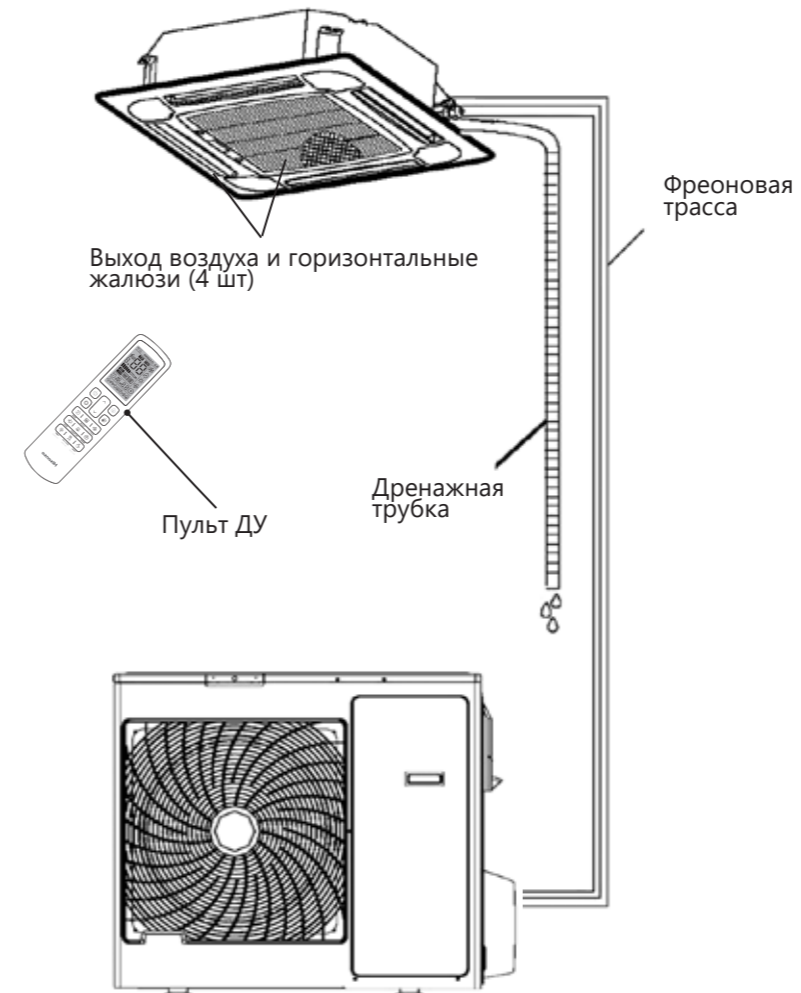
Наружный блок (типоразмер 12/18/24/36/60)
